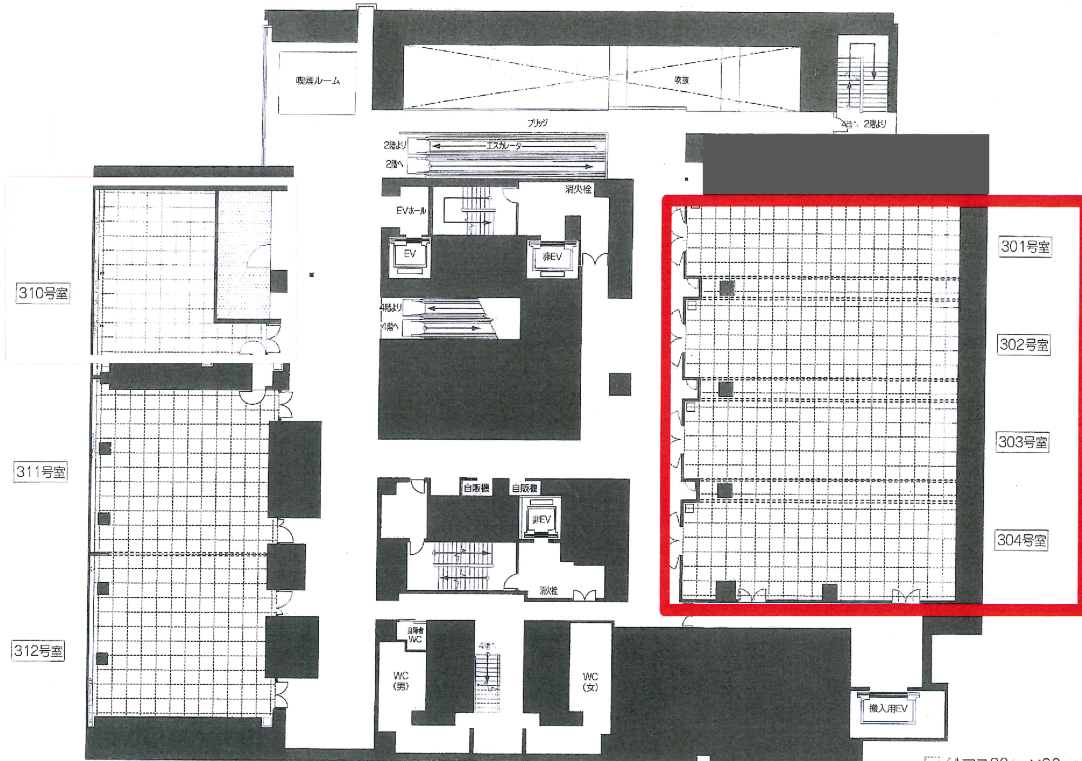
□ (1マス90cm×90cm) 1:200 3階平面図
